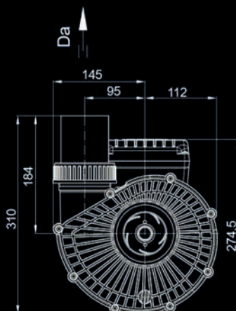
Abmessungen der PRO Flow-F und PRO Flow-D gleiche Maße, 2 Funktionen
