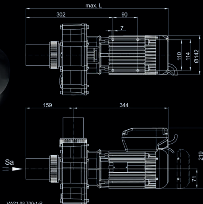
Abmessungen der PRO Flow-F und PRO Flow-D gleiche Maße, 2 Funktionen
