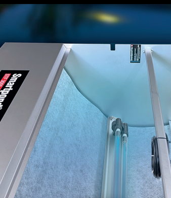
Vliesfilter STF 3000 / 500
